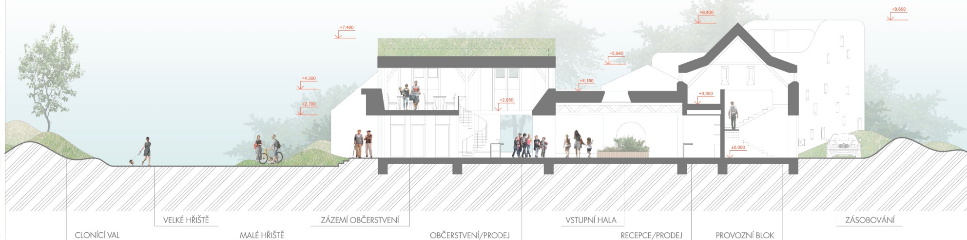
SVISLÝ ŘEZ D - D'
