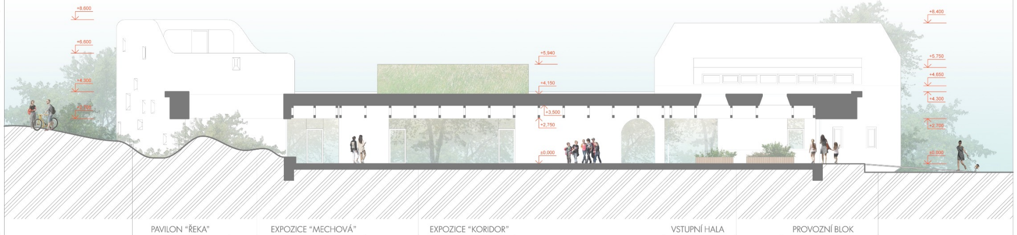
SVISLÝ ŘEZ B - B'
